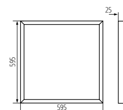
BAREV R 36W 6060
