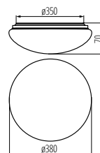
CORSO LED N 18W / 18W-SE
